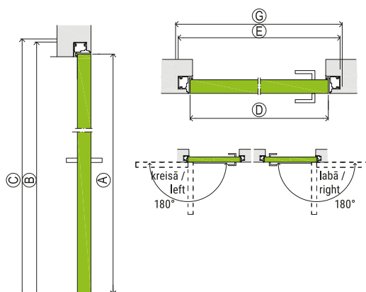
UZSTĀDĪŠANA IZMANTOJOT APMETUMU INSTALLATION WITH THE USE OF MORTAR
