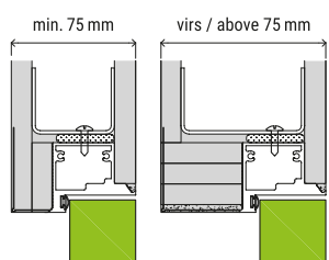
UZSTĀDĪŠANA IZMANTOJOT ĢIPSĶĀRTONA PLĀKŠNI INSTALLATION WITH THE USE OF DRYWALL
