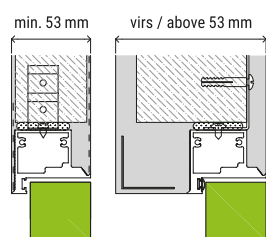
UZSTĀDĪŠANA IZMANTOJOT APMETUMU INSTALLATION WITH THE USE OF MORTAR
